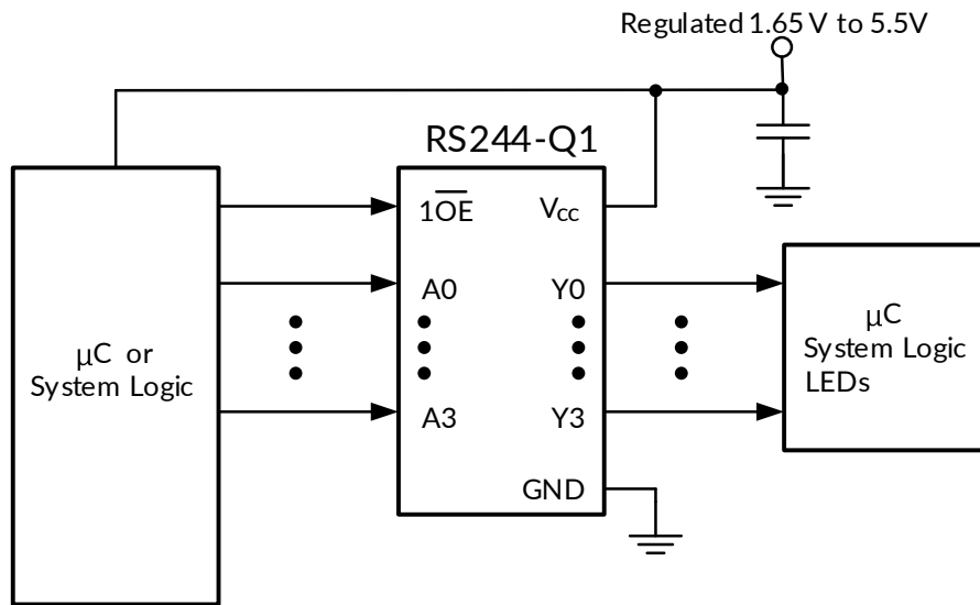
图 4. 典型应用电路
