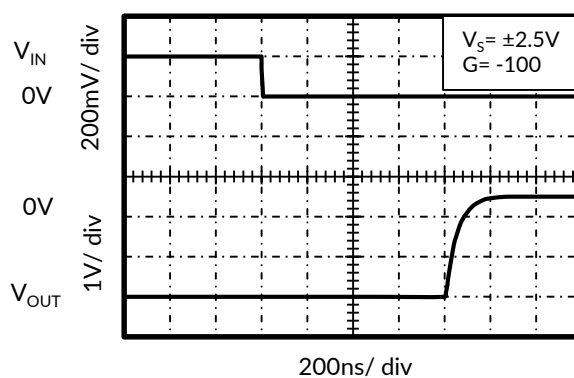
图 10. 反向过载恢复
