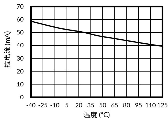
图 3. 拉电流与温度的关系
