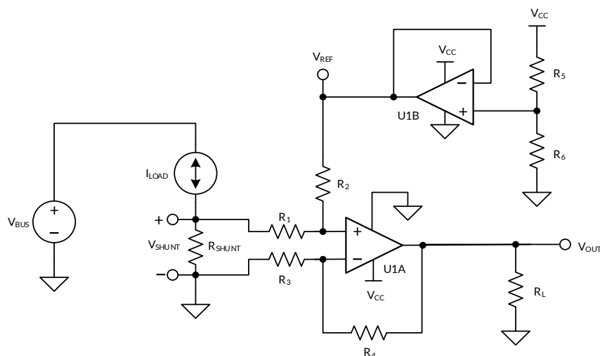
图 13. 双向电流检测应用
