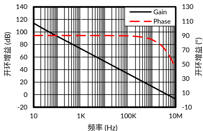
图 1. 开环增益和相位裕度与频率的关系
