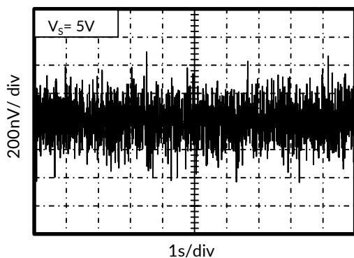
图 11. 0.1Hz ~ 10Hz 噪声
