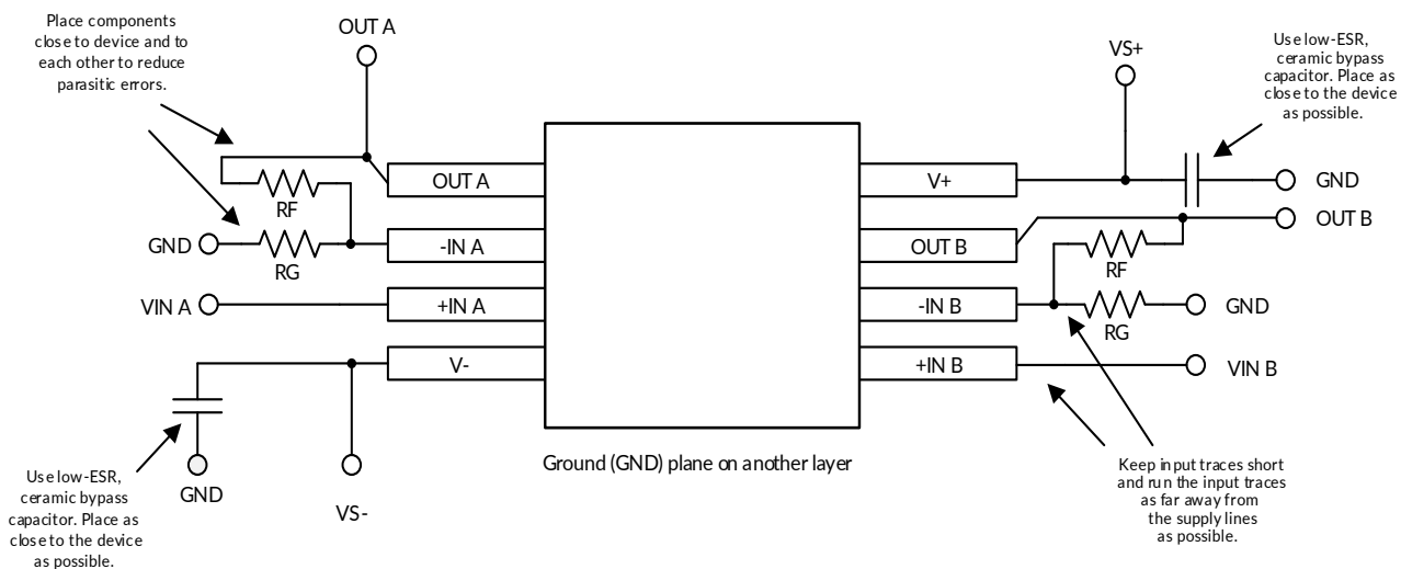
图 16. PCB 布局建议
