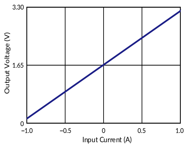
图 14. 双向电流检测电路：输出电压和输入电流的关系
