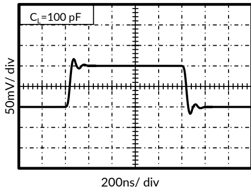
图 7. 小信号阶跃响应
