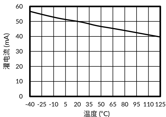
图 4. 灌电流与温度的关系
