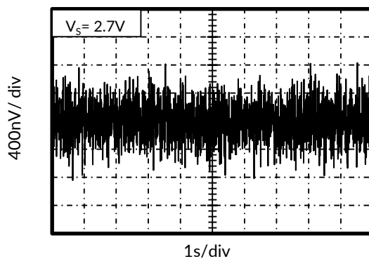
图 12. 0.1Hz ~ 10Hz 噪声
