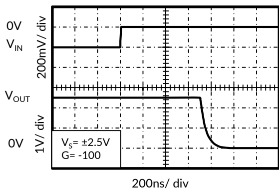
图 9. 正向过载恢复
