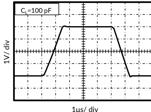
图 8. 大信号阶跃响应
